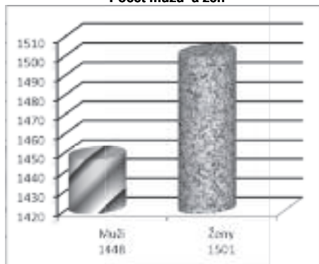
Počet mužů a žen
