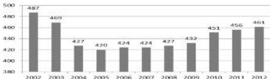
Počet dětí do 15 let
