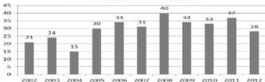
Počet dětí do 15 let
